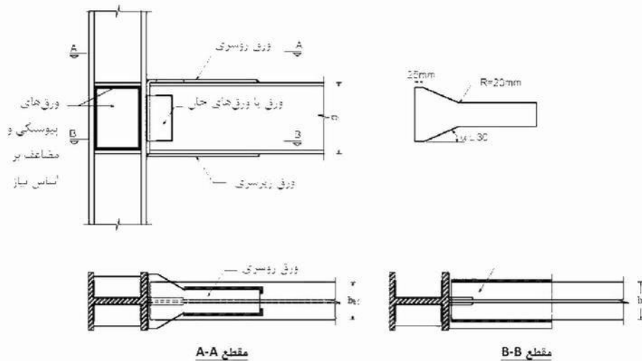
شکل ۳-۱۰-۷-۶: اتصال گیردار جوشی به کمک ورق‌های روسری و زیرسری (WFP)
