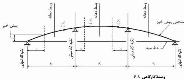
نمای جانی پیش‌نصب تیر
