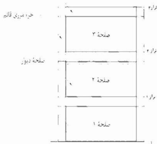
شکل ۱۰-۳-۴-۵-۱: پیکر بندی دیوار برشی فولادی ویژه
