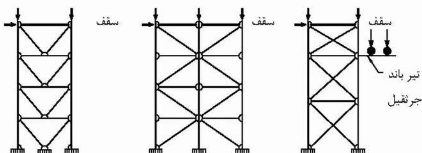
مهاربند چند ردیفی از نوع ۷ مهاربند چند ردیفی دو دهانه مهاربند چند ردیفی ضربدری
