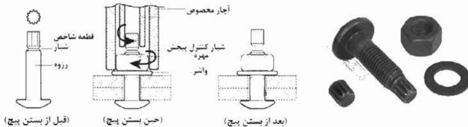
شکل ۱۰-۴-۵: پیچ کشش-کنترل (TC Bolt)
