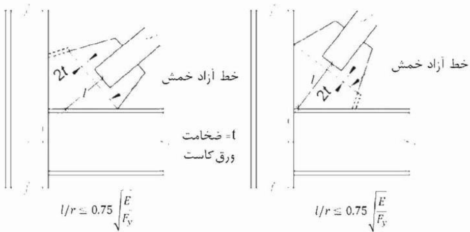
شکل ۳-۱۰-۲-۴-۳-۱۰: سازگاری ورق اتصال (ورق کاست) با کمانش خارج از صفحه عضو مهاربندی
