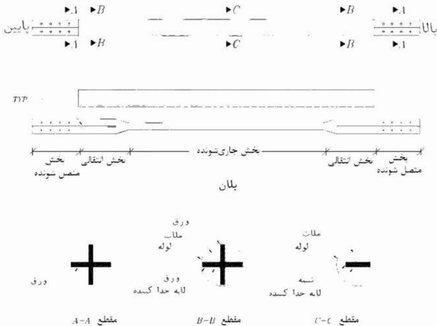
شکل ۳-۱۰-۴-۴-۱: نمونه‌ای از اجزای یک مهاربند کمانش تاب
