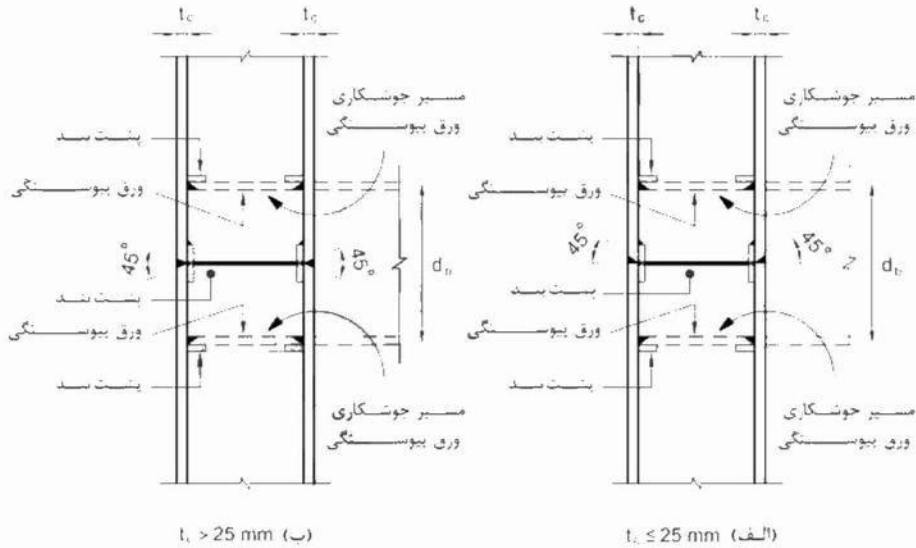
شکل ۱۰-۳-۲-۲: گزینه دیگر موقعیت وصله کارخانه‌ای ستون‌ها
