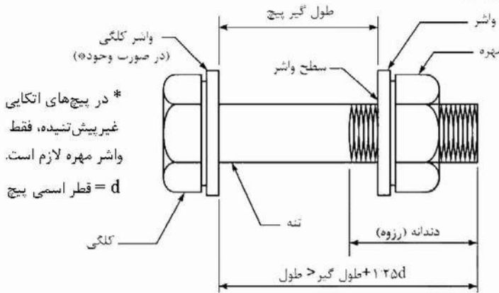
شکل ۳-۴-۱۰: اجزای مختلف پیچ و مهره
