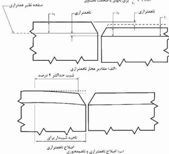
شکل ۱۰-۴-۹: ناهمترایی و اصلاح آن
