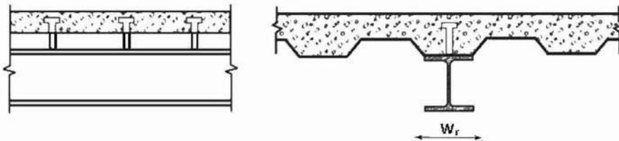
شکل ۸-۸-۲-۱۰: عرشه فولادی که کنگره‌های آن موازی با محور طولی تیر است
