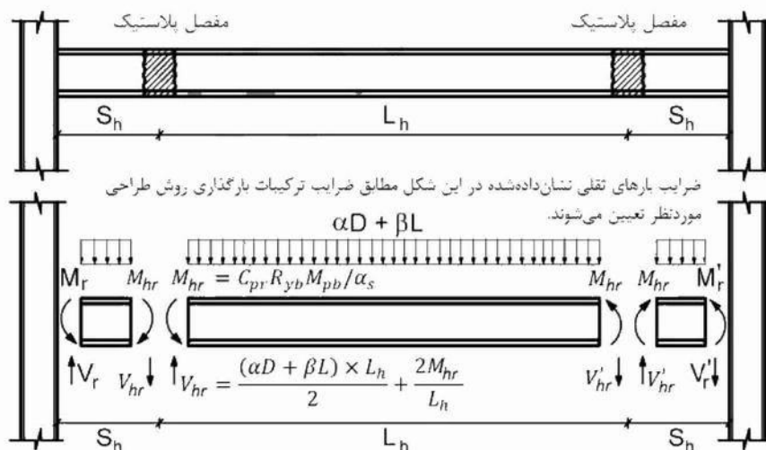
شکل ۱۰-۳-۳-۱: نمودار پیکره آزاد تیرهای برابر لرزه‌ای در قاب‌های خمشی ویژه
