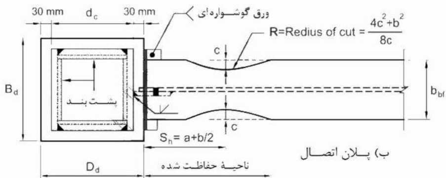
شکل ۱۰-۳-۷-۱۲: اتصال گیردار تیر با مقطع کاهش یافته و دیافراگم عبوری از ستون در قاب‌های خمشی متوسط
