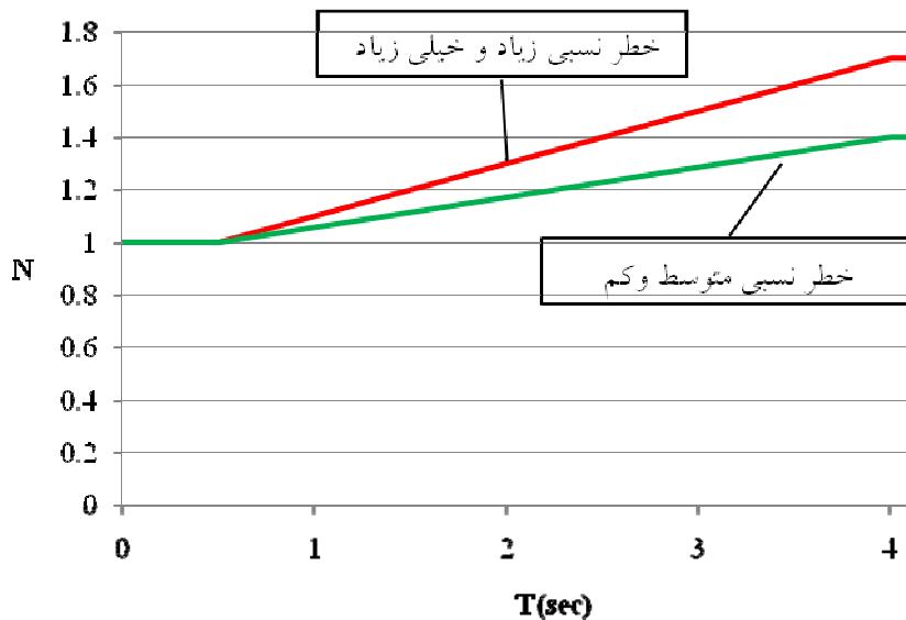
شکل ۲-۲ ضریب اصلاح طیف، N ، خاک نوع II
