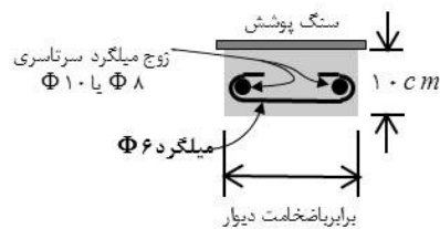
شکل ۱۶-۷ جزئیات مهار جان پناه
