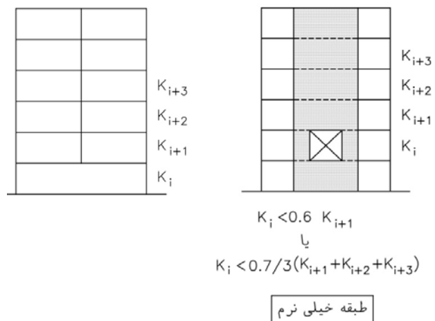
ث - نامنظمی سختی جانبی
